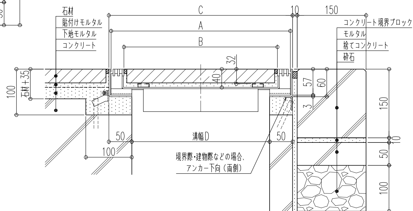
施工参考図
